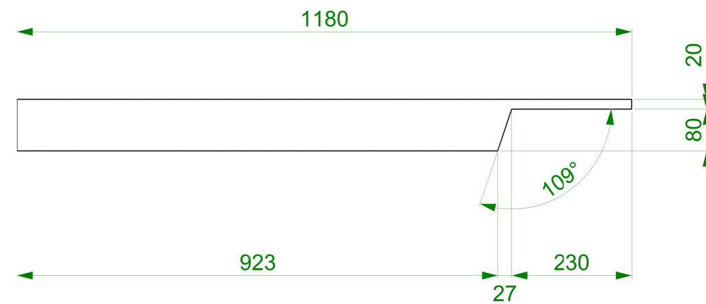
Elévation frontale
